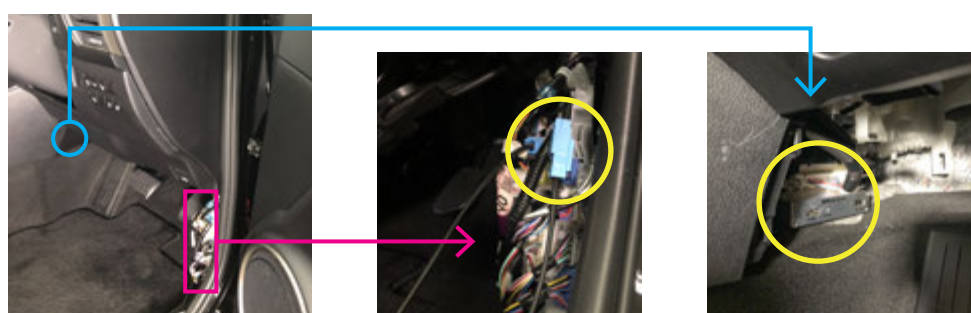
GVIFケーブル接続位置 (運転席キック内)
